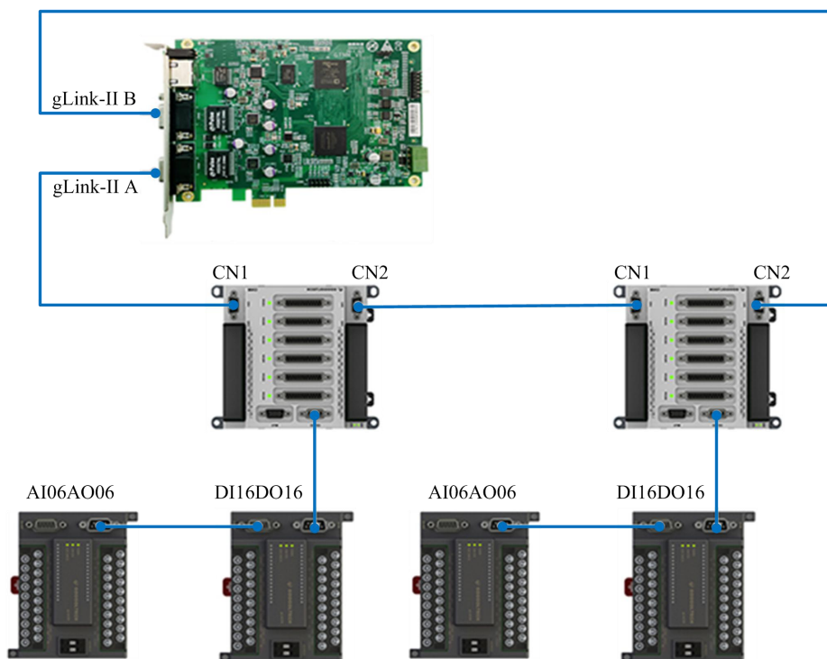
图 1 GXN 系列产品扩展模块连接示意图
