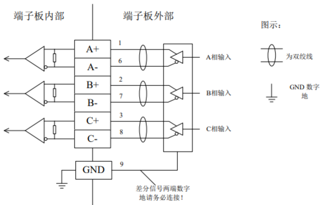
图 3-8: 辅助编码器差分电路图
