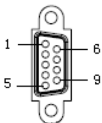
图 3-7 端子板辅助编码器接口 (CN13 ENC) 接口引脚号说明
