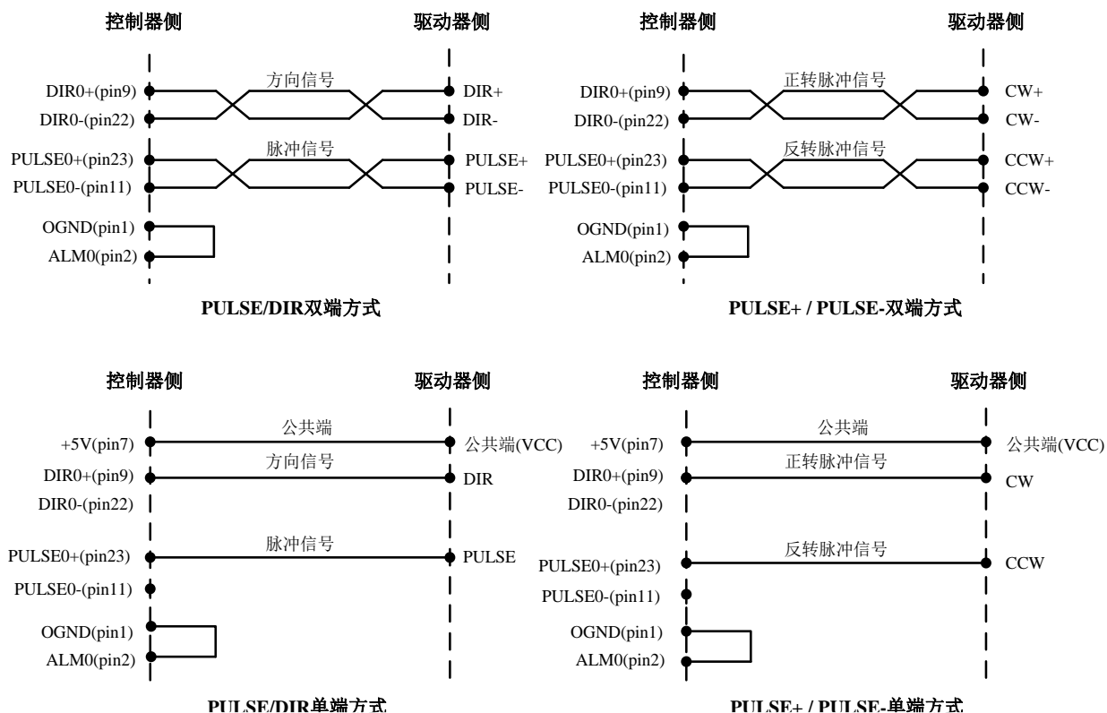
图 3-13 脉冲量输出信号连接图
