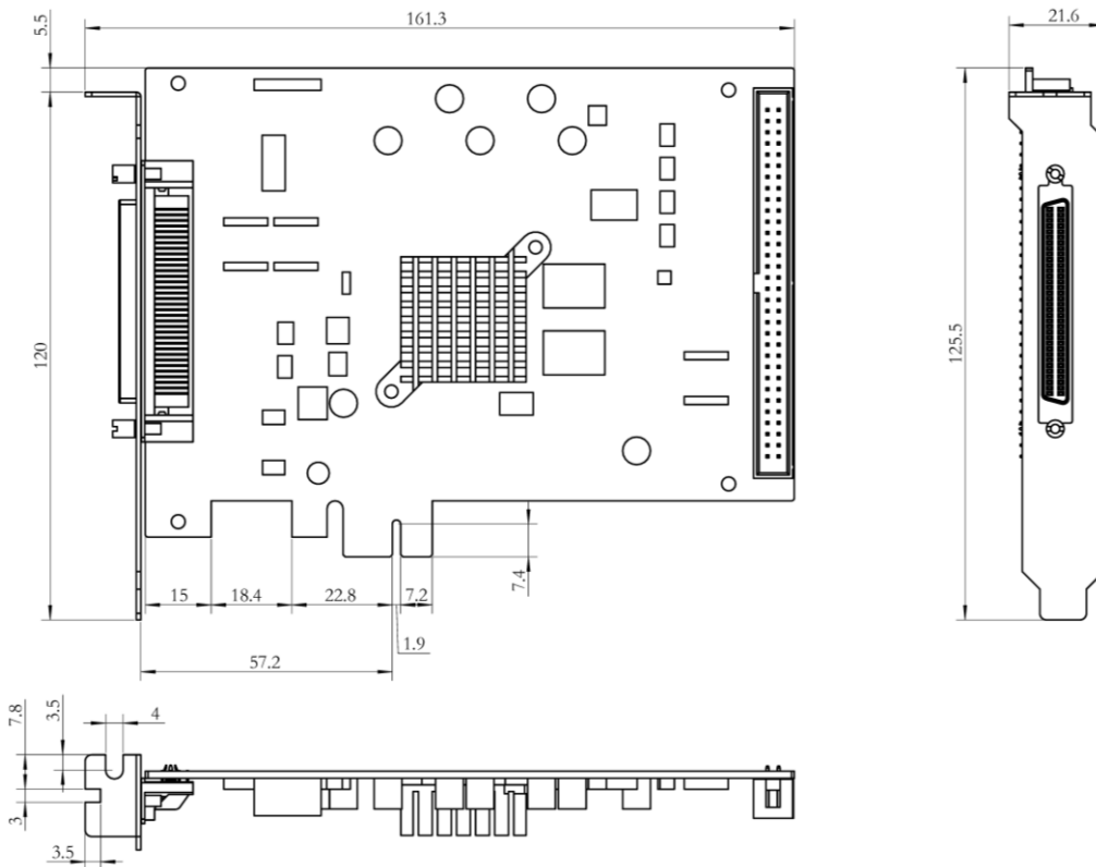
图 6-22 GTS14 轴运动控制器 (主卡) 尺寸图 单位 (mm)
