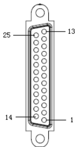
图 3-1 端子板 CN1-CN8 接口引脚号说明
