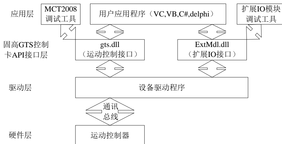
图 4-2 软件架构图
