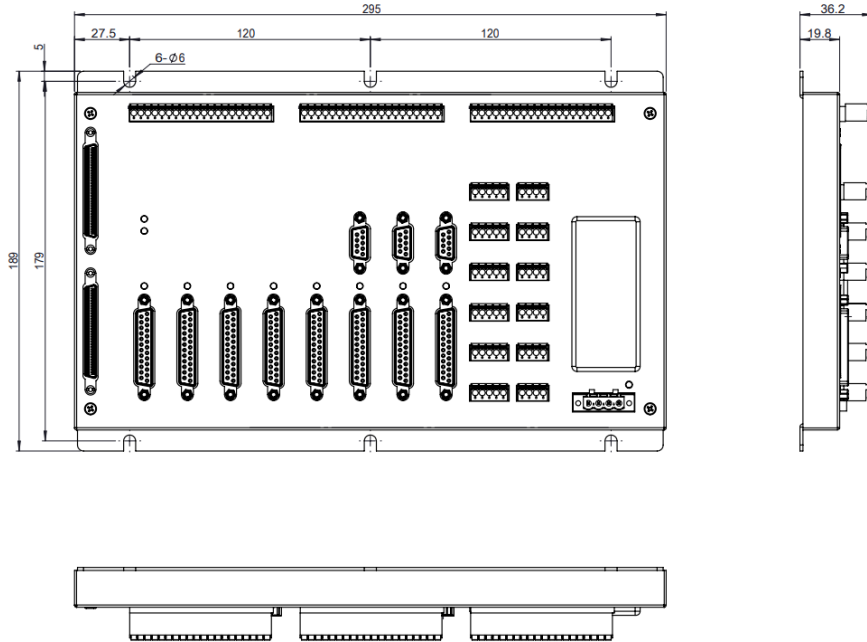
图 6-21 GTS14 轴端子板机械尺寸图 单位 (mm)
