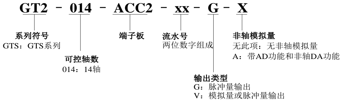
图 1-2 端子板型号说明
