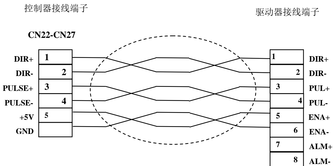
图 6-20 雷赛 DM-S/DM V3.0 系列升级型步进电机驱动器接线
