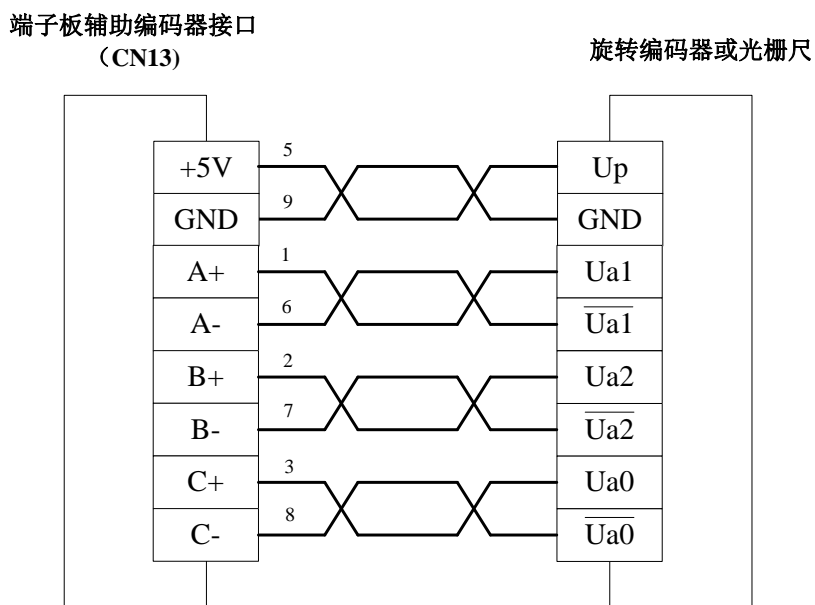
图 5-4 接海德汉旋转编码器
