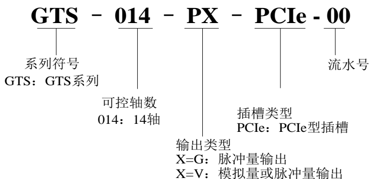
图 1-1 GTS-PCIe 标准版 14 轴控制器型号说明
