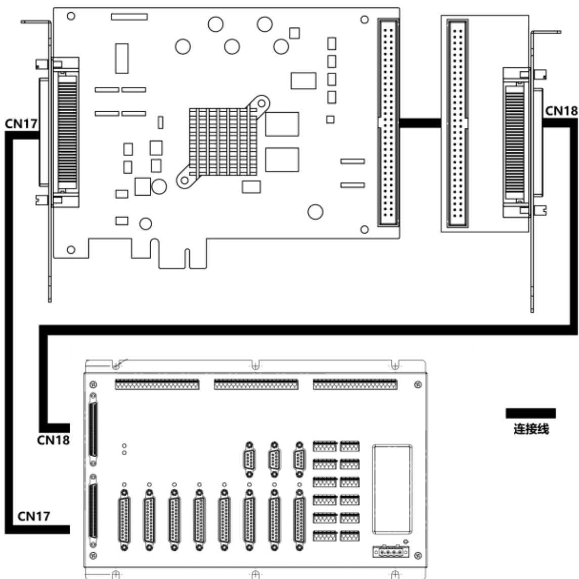
图 2-10 运动控制器与 14 轴端子板连接示意图
