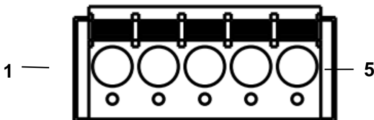
图 3-11 端子板 9-14 轴步进轴电机控制信号接口引脚说明 CN22-CN27 为第 9-14 轴步进电机控制信号端口，其引脚和信号对应关系见表所示
