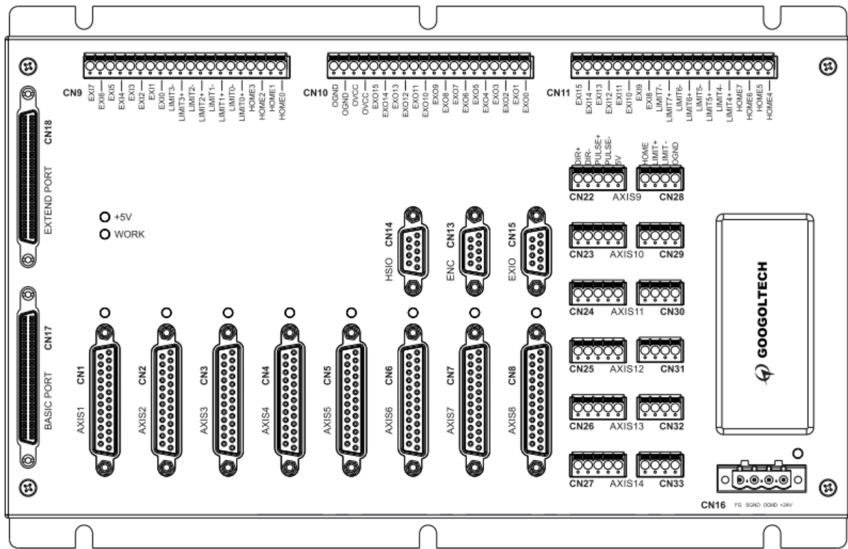
图 1-5 14 轴端子板俯视图
