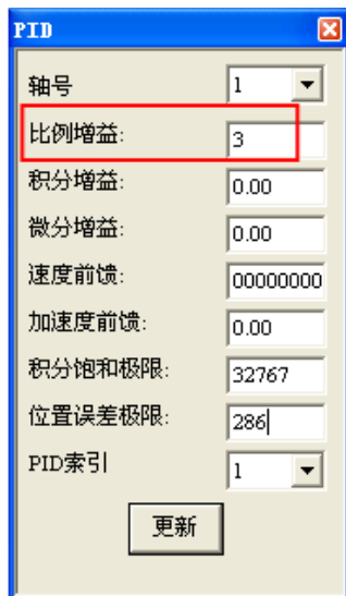
图 4-11 PID 设置选项
