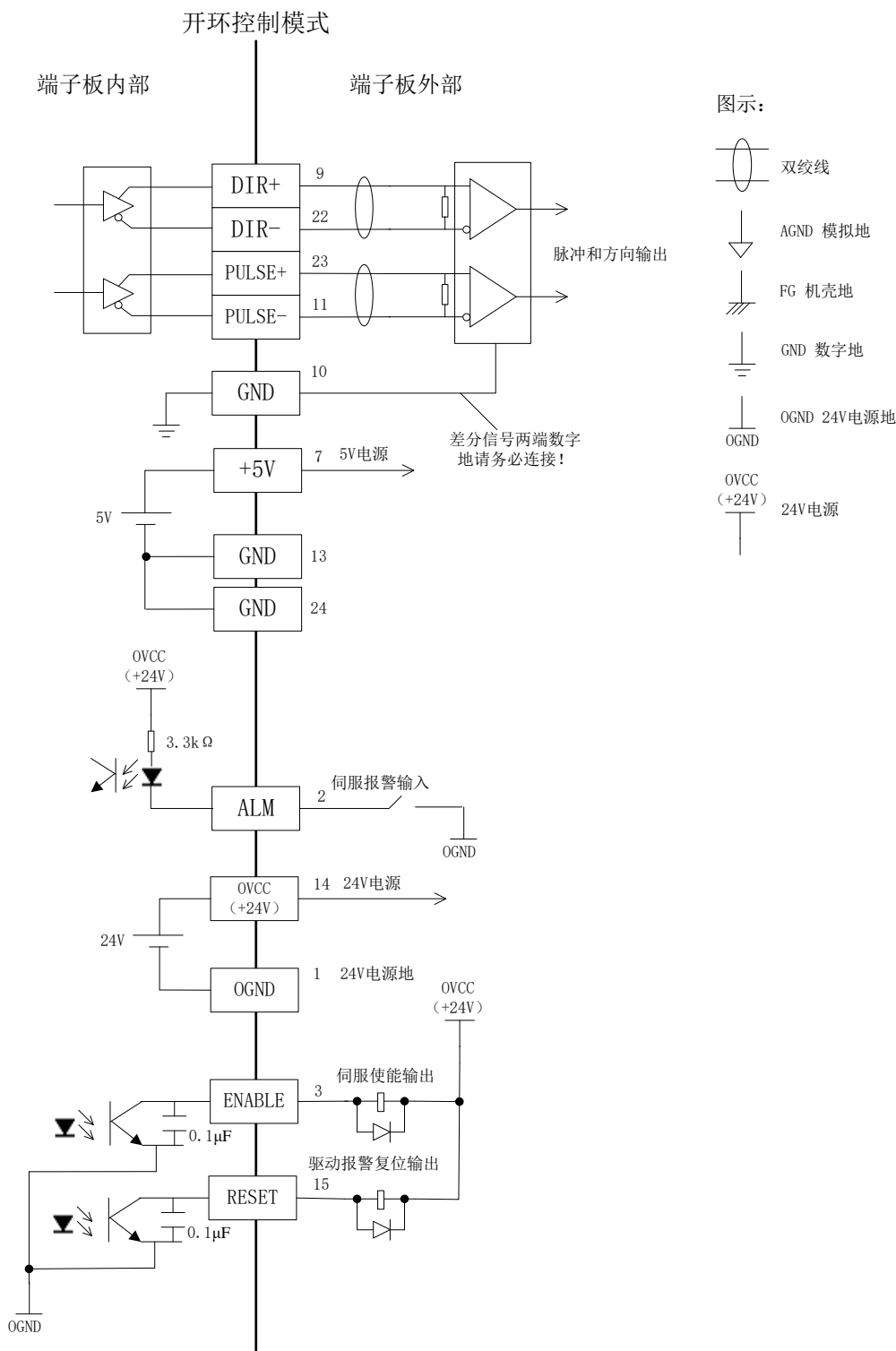
图 3-12 开环控制模式下轴信号接口（CN1-CN8）内部电路
