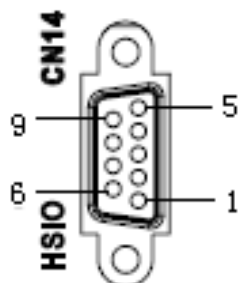
图 3-5 端子板 CN14 HSIO 接口引脚号说明
