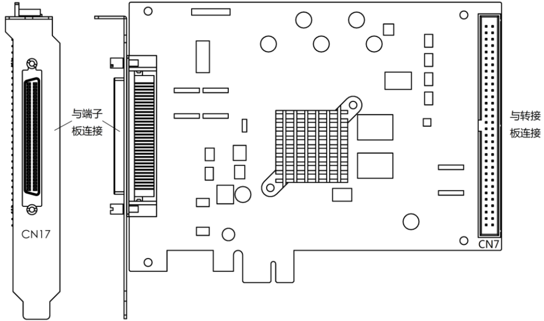
图 1-3 GTS-PCIe 版 14 轴控制器的侧视图（左）和俯视图
