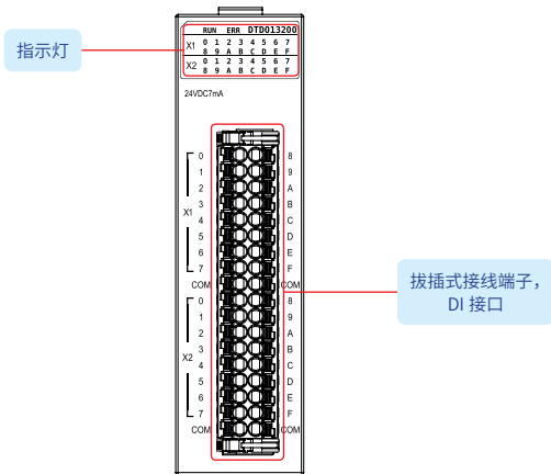
LIMIT/HOME 专用数字 IO 模块
