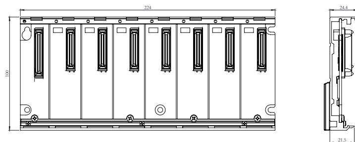
七槽专用基板模块
