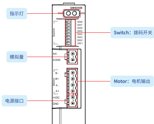
GMSD556 单轴步进驱动器模块
