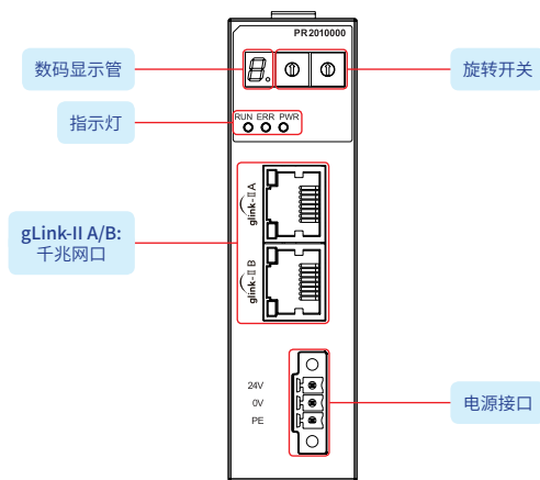
通讯及电源模块
