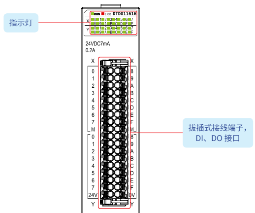
通用数字 IO 模块 (16DI&16DO)
