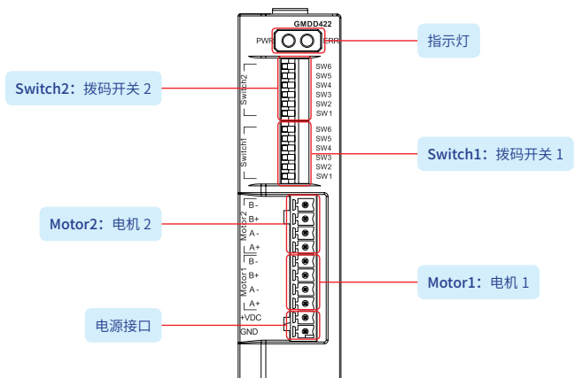
GMDD422 双轴步进驱动器模块
