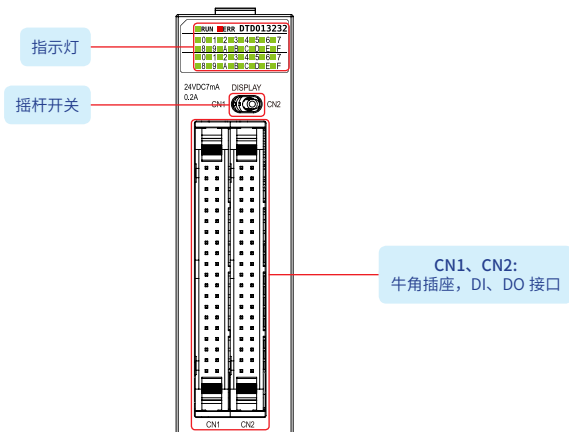
通用数字 IO 模块 (32DI&32DO)
