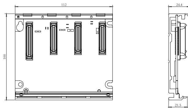
三槽专用基板模块
