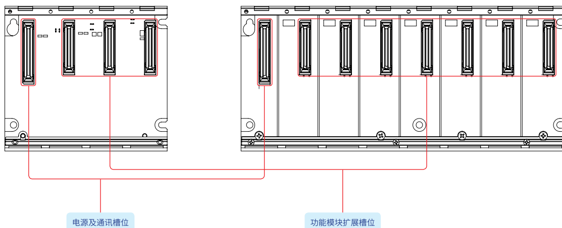
三槽 / 七槽专用基板模块
