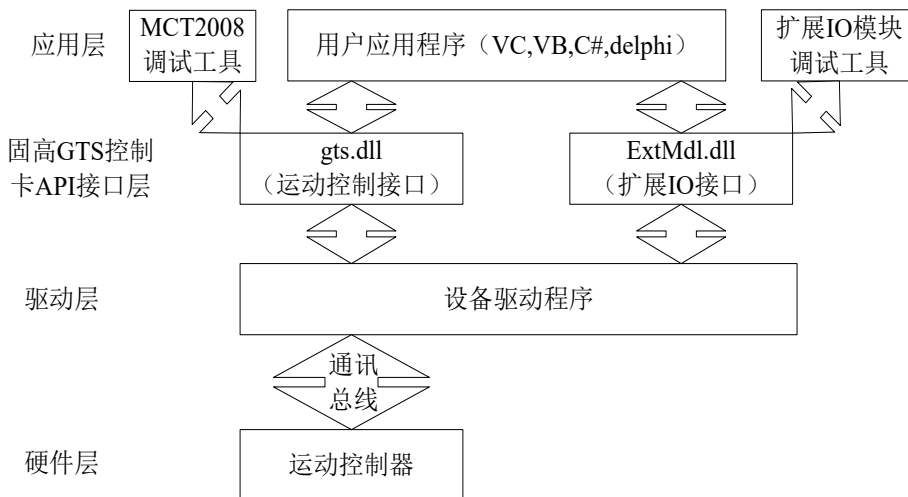
图 4-2 软件架构图
