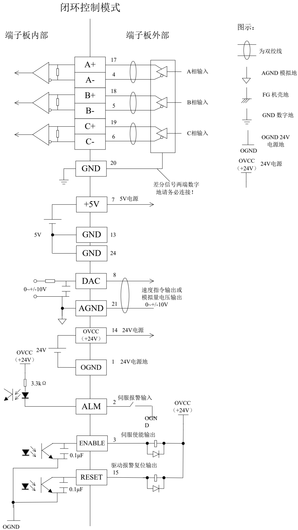
图 3-11 闭环控制模式下轴信号接口(CN1-CN8)内部电路
