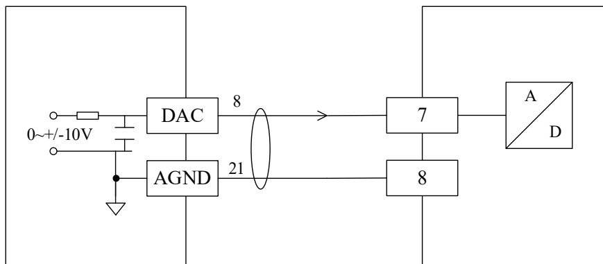
图 5-1 模拟量控制变频器接线方法
