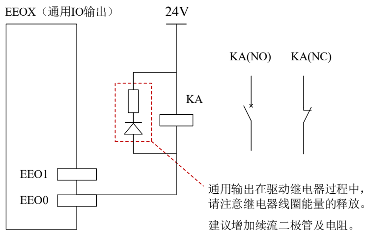
图 5-3 通用输出接继电器
