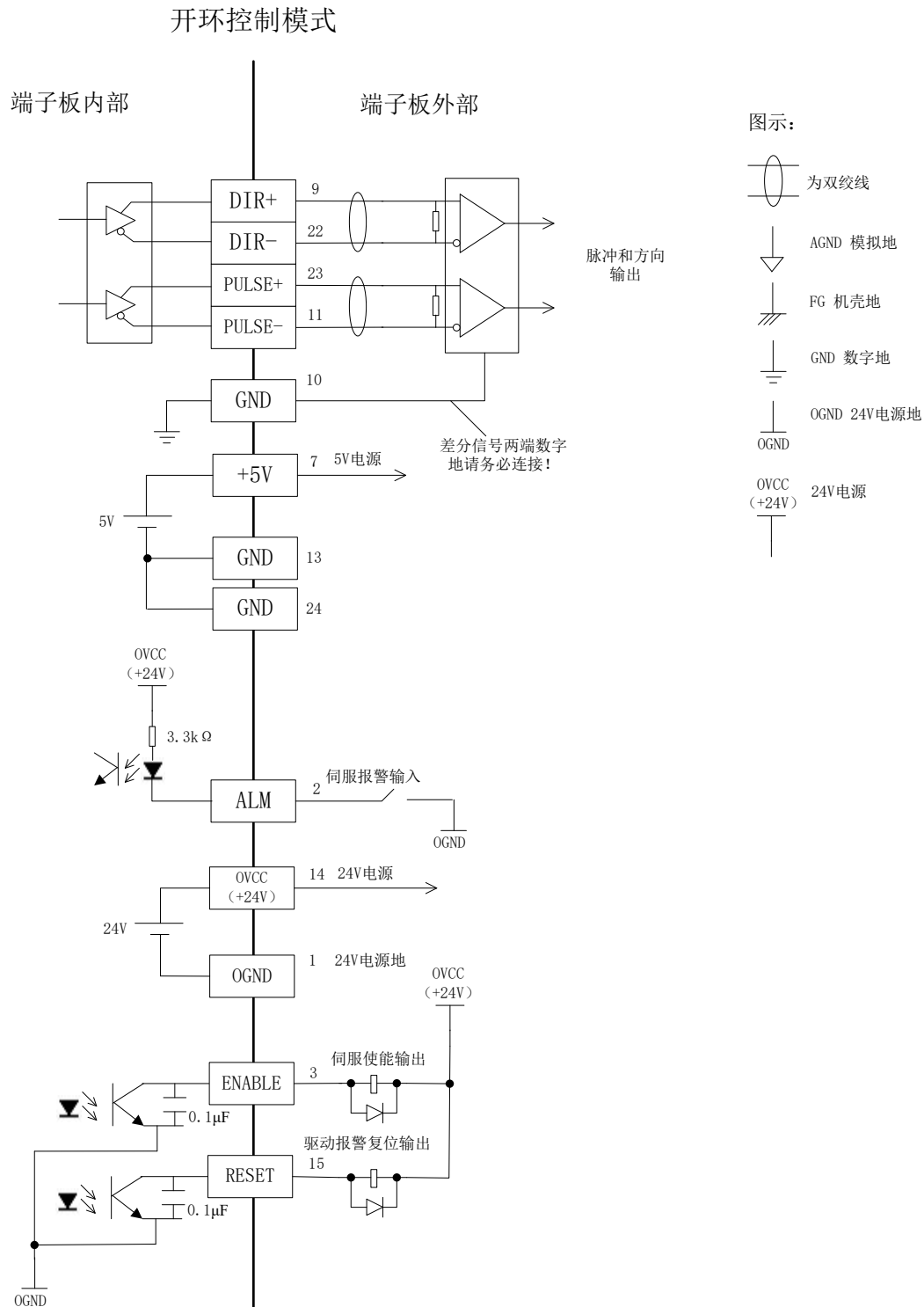
图 3-8 开环控制模式下轴信号接口（CN1-CN8）内部电路
