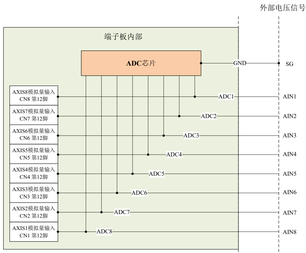
图 3-6 端子板模拟量输入内部电路示意图
