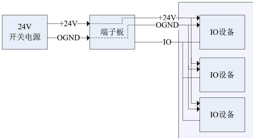
图 6-1 端子板供电示意图
