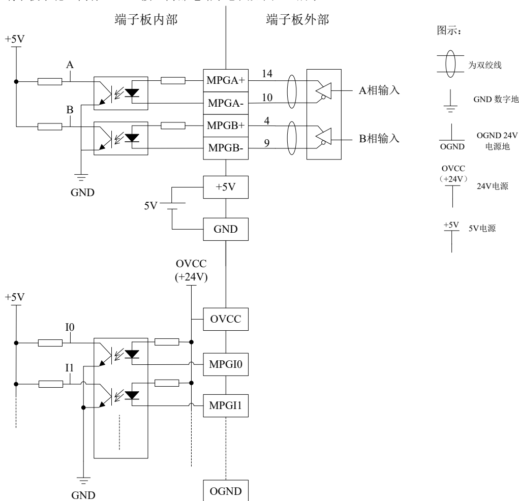
图 3-2 手轮 MPG 接口内部电路示意图
