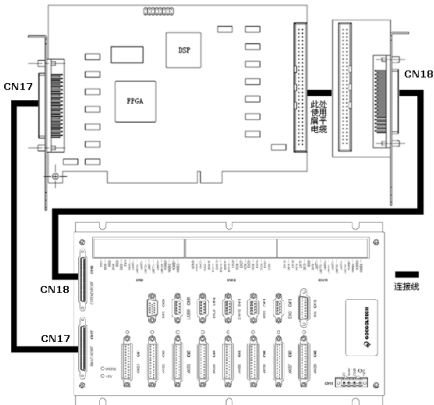
图 2-20 运动控制器与 8 轴端子板连接示意图
