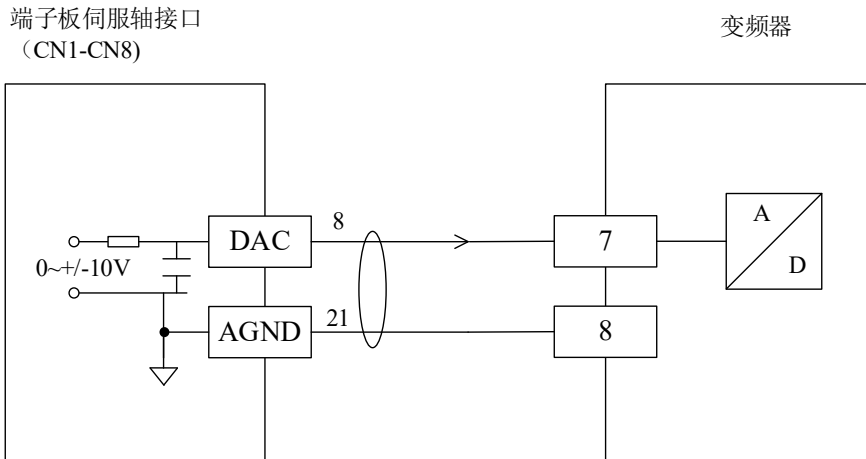
图 5-1 模拟量控制变频器接线方法
