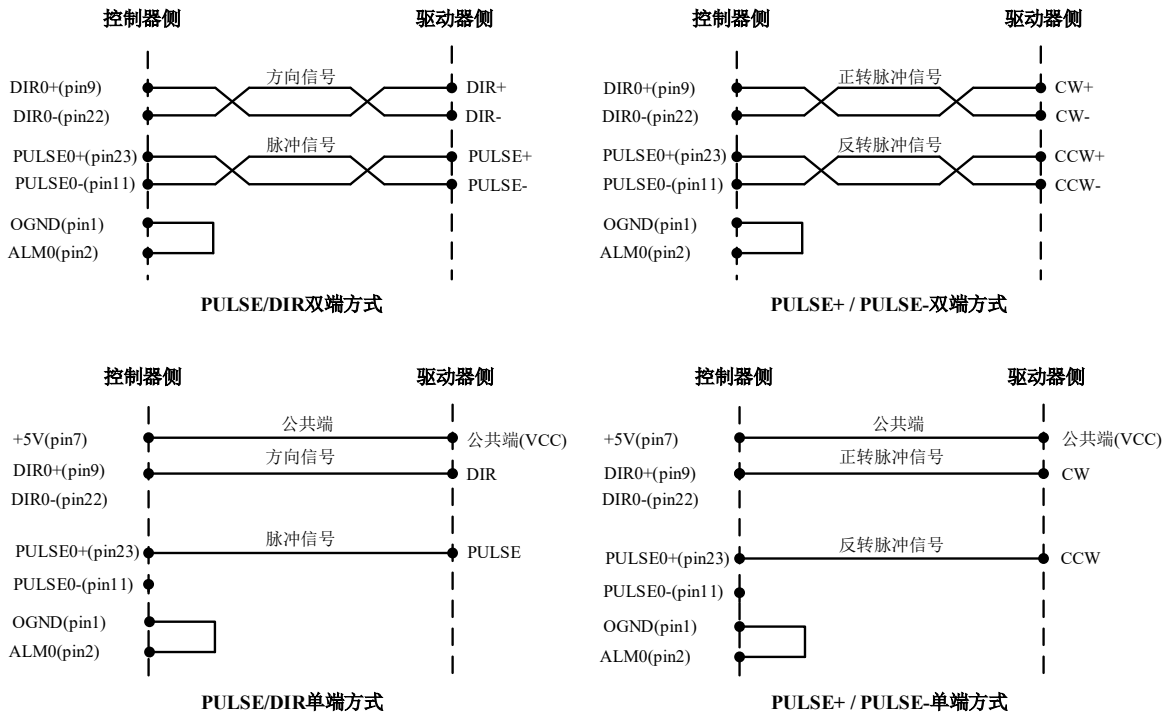
图 3-4 脉冲量输出信号连接图
