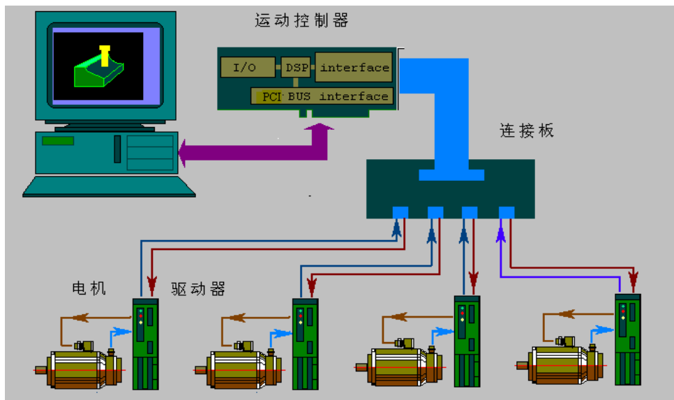
图 2-22 典型系统连接图
