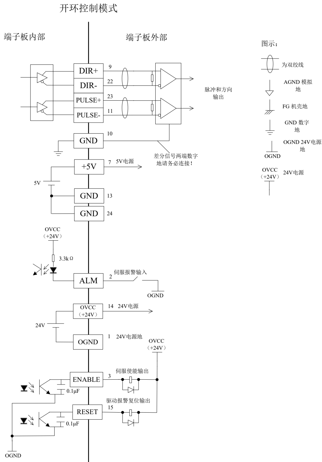
图 3-3 开环控制模式下轴信号接口（CN1-CN8）内部电路
