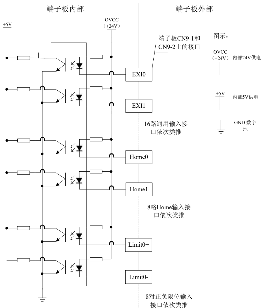
图 3-4 端子板通用输入，HOME 输入，LIMIT 输入信号内部电路示意图
