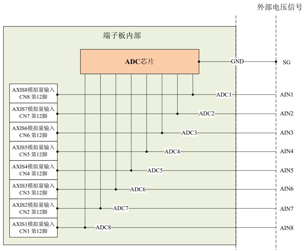
图 3-1 端子板模拟量输入内部电路示意图
