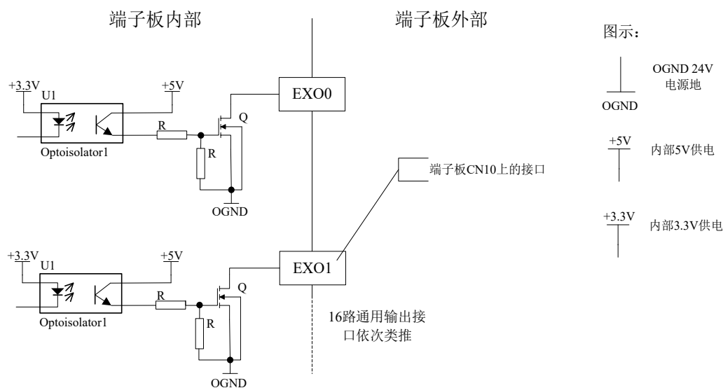
图 3-5 端子板通用数字输出信号内部电路示意图
