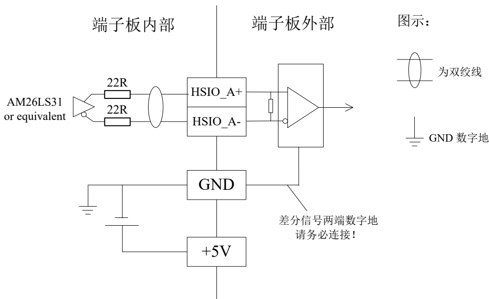
图 3-9 端子板 HSIO 接口（CN14）内部电路
