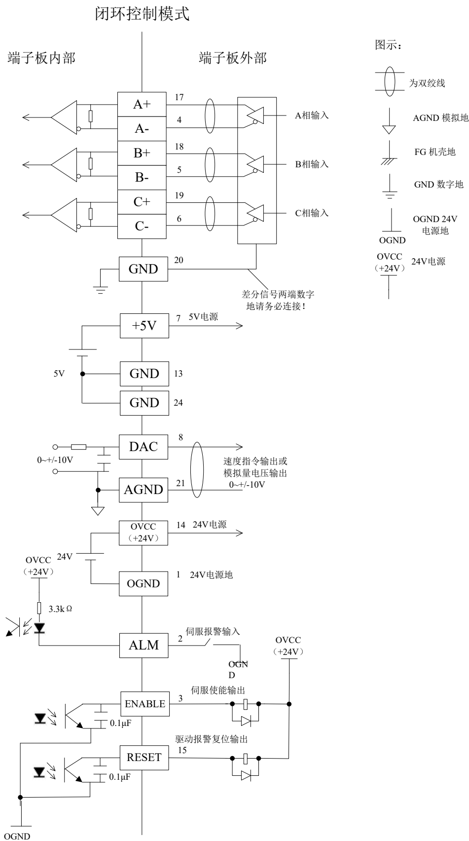
图 3-6 闭环控制模式下轴信号接口(CN1-CN8)内部电路
