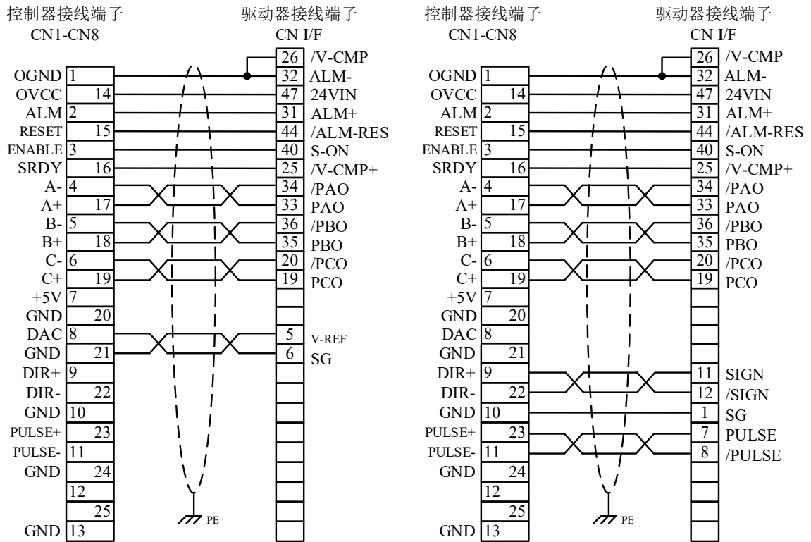
图 6-10 安川Σ-7系列驱动器速度&力矩控制方式(a)接线/位置控制方式(b)接线
