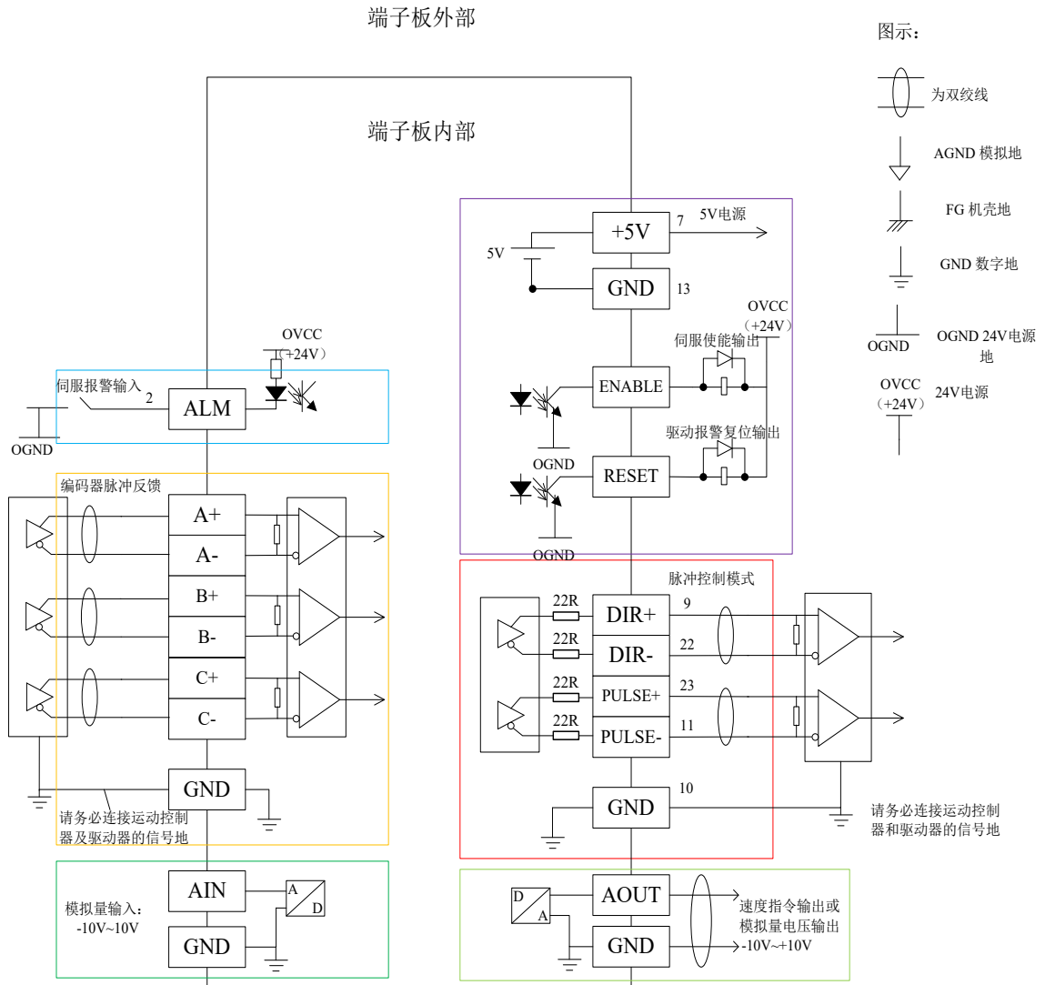
图 3-3 端子板轴信号接口内部电路
