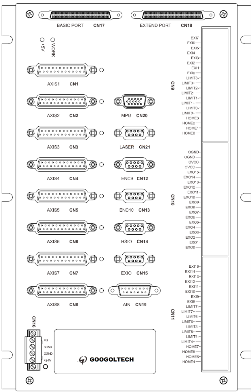
图 1-5 8 轴端子板俯视图
