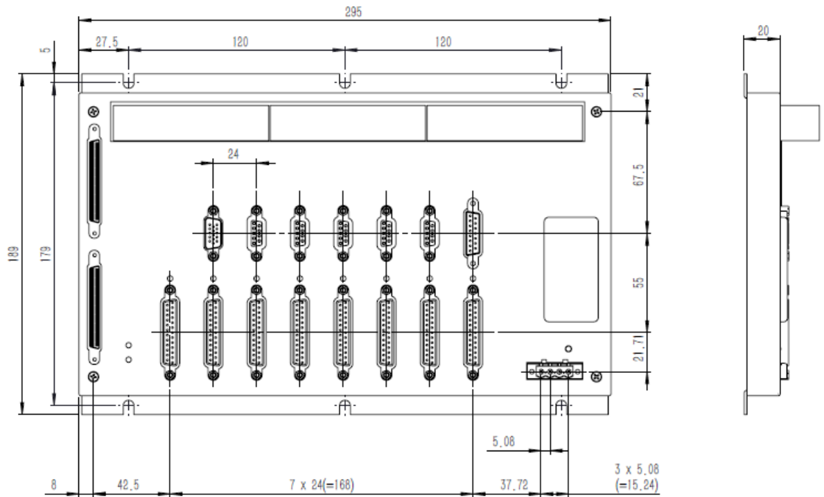
图 6-20 8 轴端子板机械尺寸图 单位 (mm)
