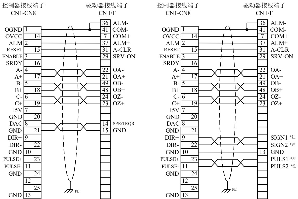
图 6-2 松下 Panasonic MSDA 系列驱动器速度控制方式(a)/位置控制方式(b)接线
