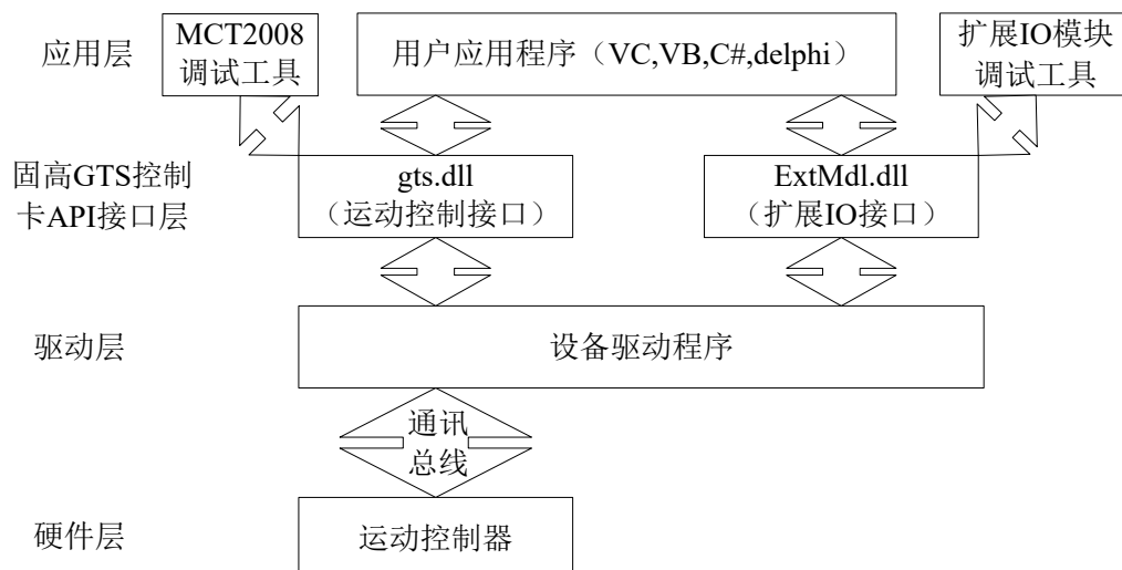
图 4-2 软件架构图
