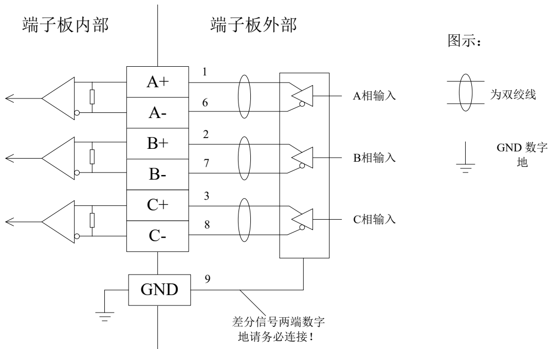
图 3-7 端子板辅助编码器接口（CN12、CN13）内部电路
