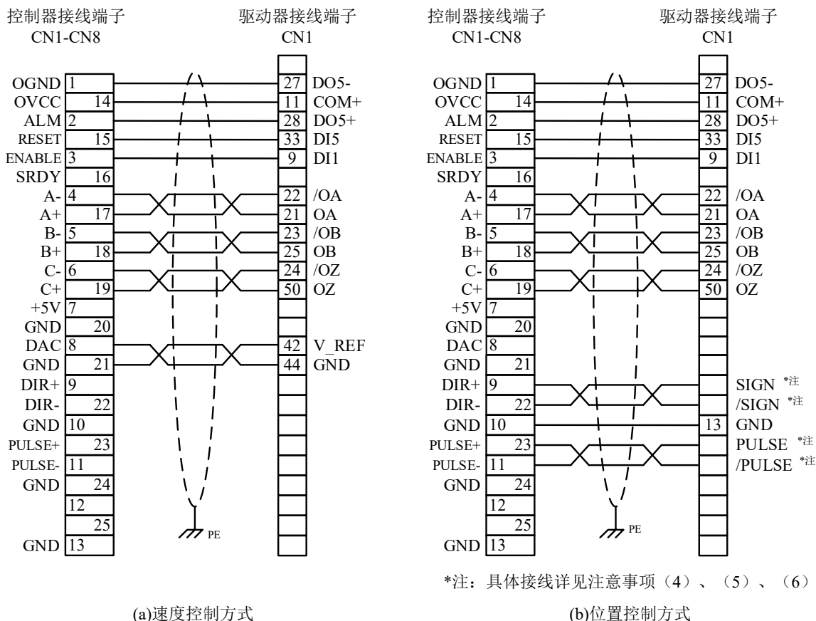
图 6-15 台达 ASDA-A2 系列驱动器速度控制方式(a)/位置控制方式(b)接线
