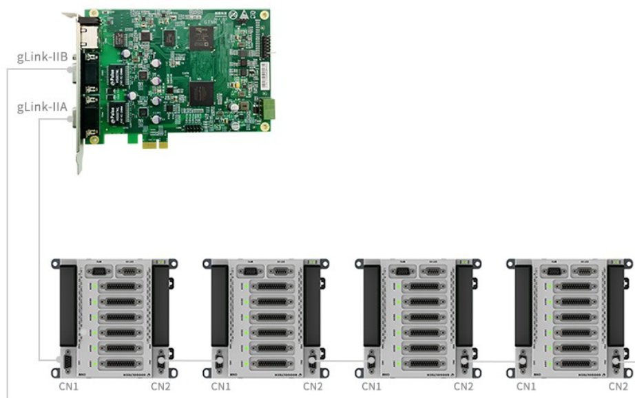
图 2-10 运动控制器与 6 轴端子板连接示意图
