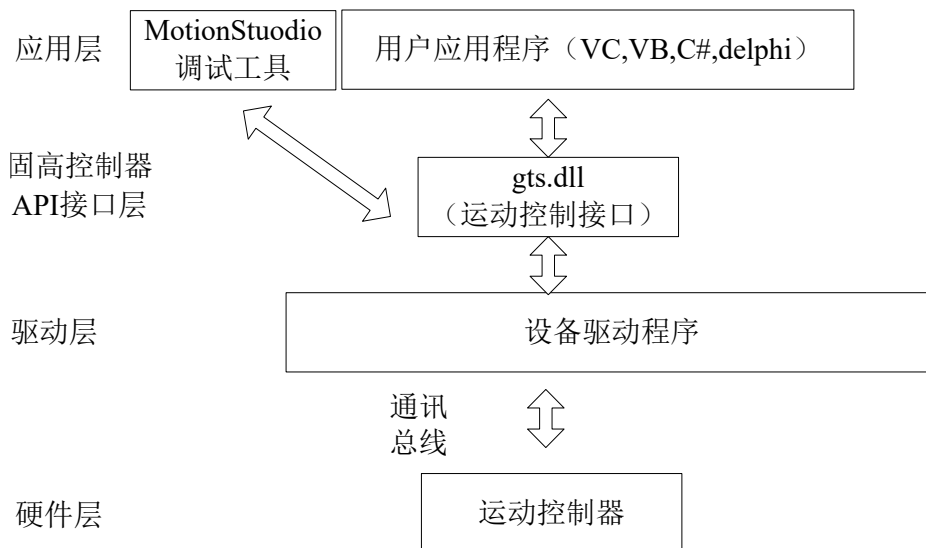
图 2-13 系统架构图
