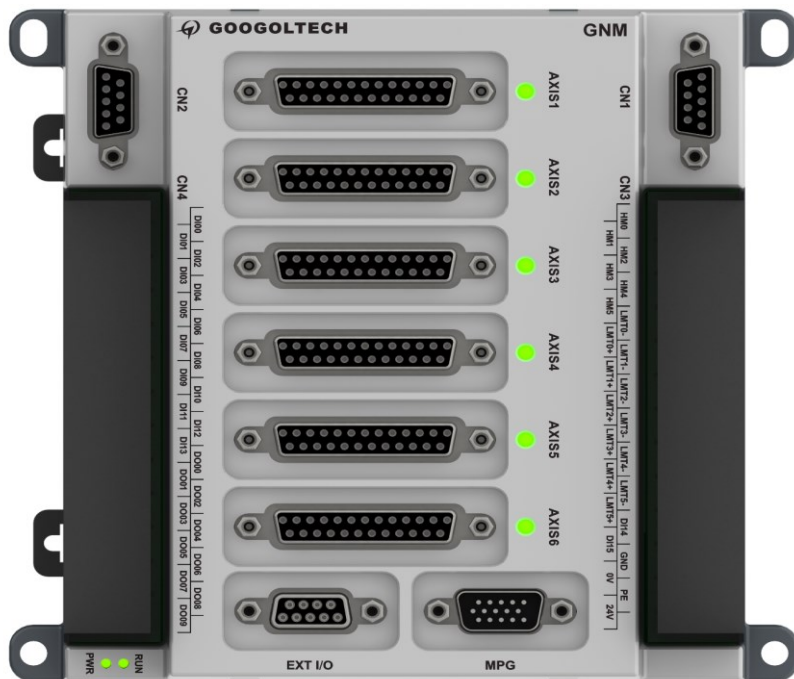
图 1-5 GNM-601-A00 端子板俯视图
