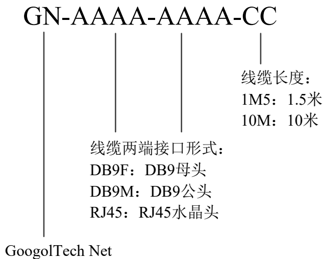
图 1-3 线缆型号说明
