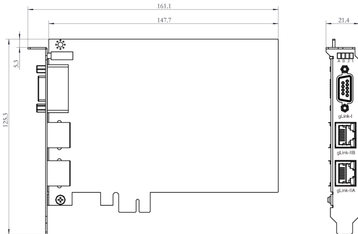
图 1-4 GSN-A00 控制器的侧视图（右）和俯视图
